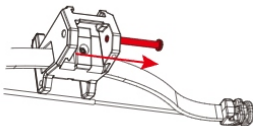
Schnellverschlussstifte
